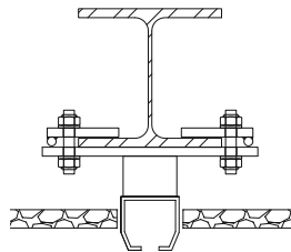
Einbausituation bei einer abgehängten Decke mit vorab montiertem Stahlträger.
